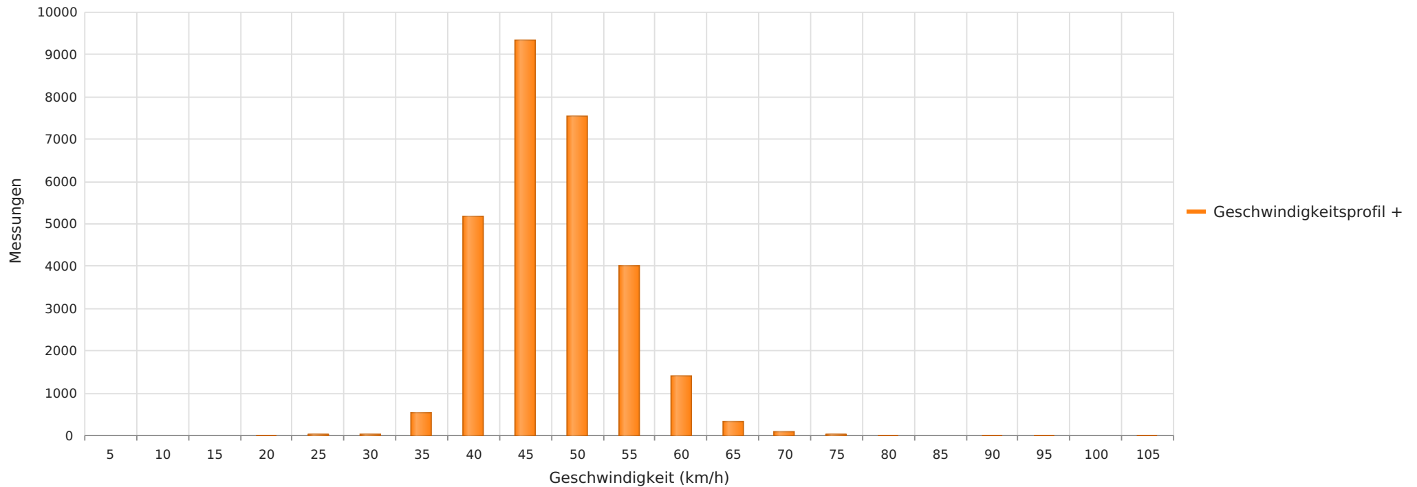
Dresdner Straße (S179), Reichenberg, Fahrtrichtung Dresden Höhe Kirchweg Anzahl der Messwerte vs. Geschwindigkeit
